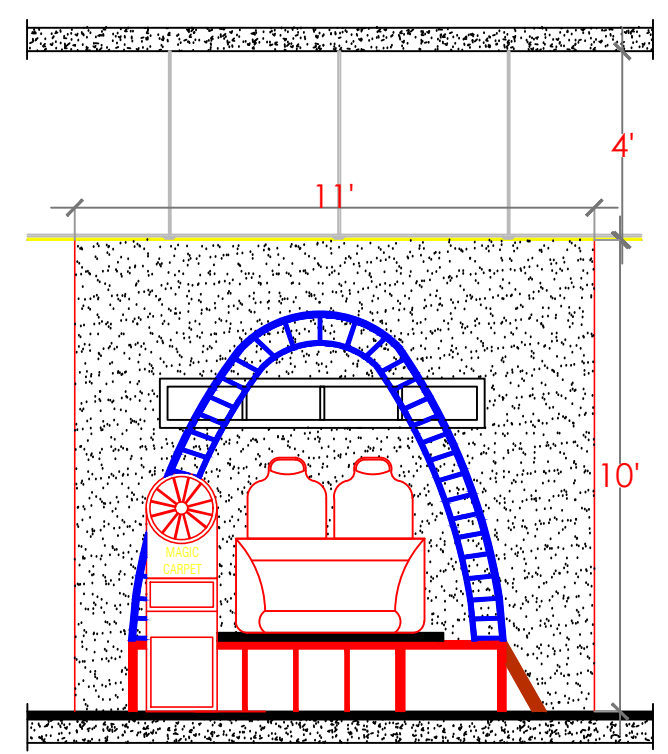
SECTION - A1
